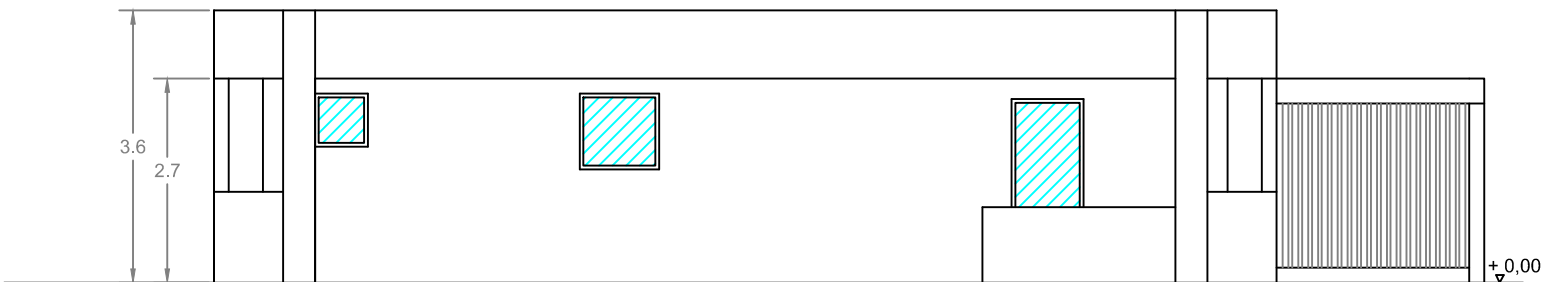
PROSPETTO OVEST
