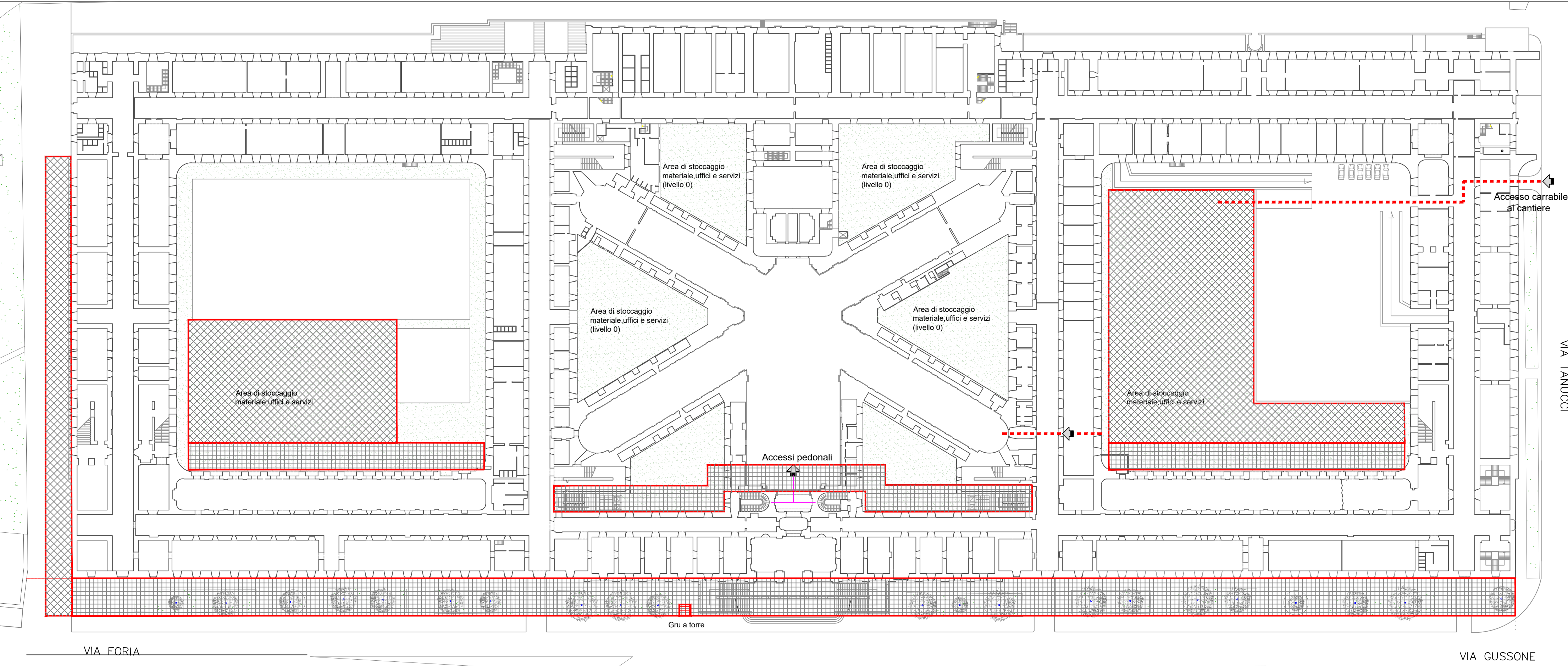
PIANTA LIVELLO 0 Planimetria con indicazione delle aree di cantiere
