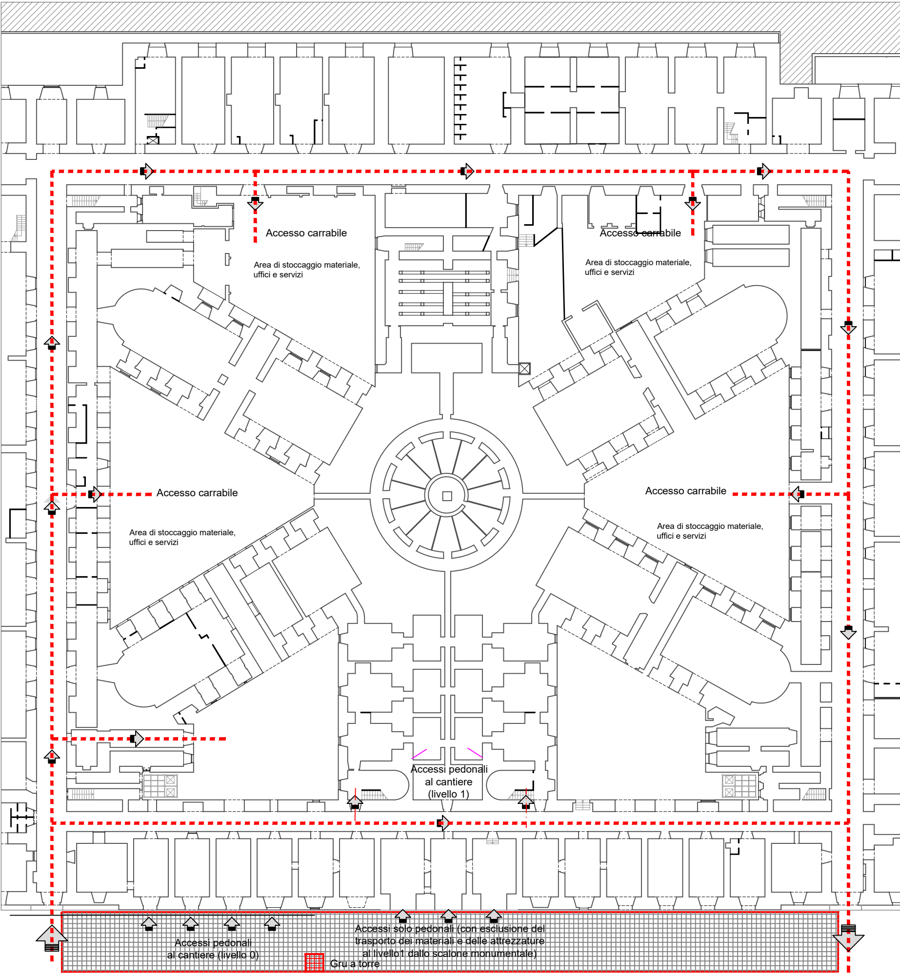
PIANTA PIANO SEMINTERRATO (LIVELLO 0) PIANTA PIANO SEMINTERRATO (LIVELLO 0) Planimetria con indicazione dei sensi di percorrenza carrabile interna al cantiere e localizzazione dei principali percorsi pedonali
