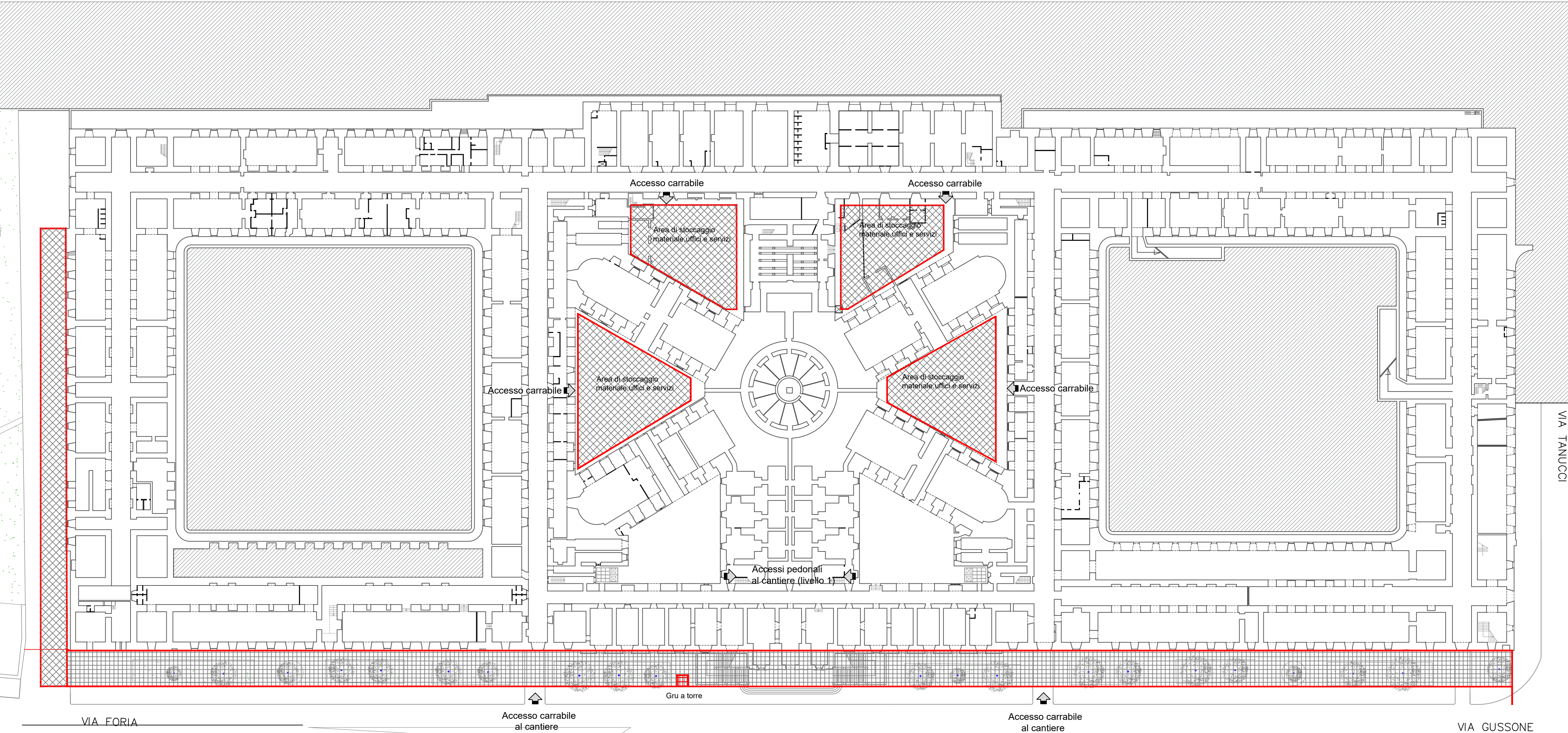
PIANTA LIVELLO 0 Planimetria con indicazione delle aree di cantiere
